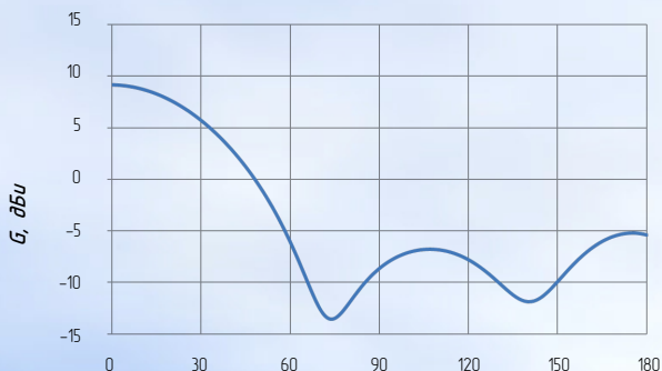
Диаграмма направленности в вертикальной плоскости
