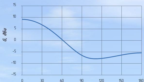
Диаграмма направленности в горизонтальной плоскости
